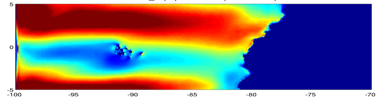
MLDR10_3 (m) - erai70c (2000-2007)
