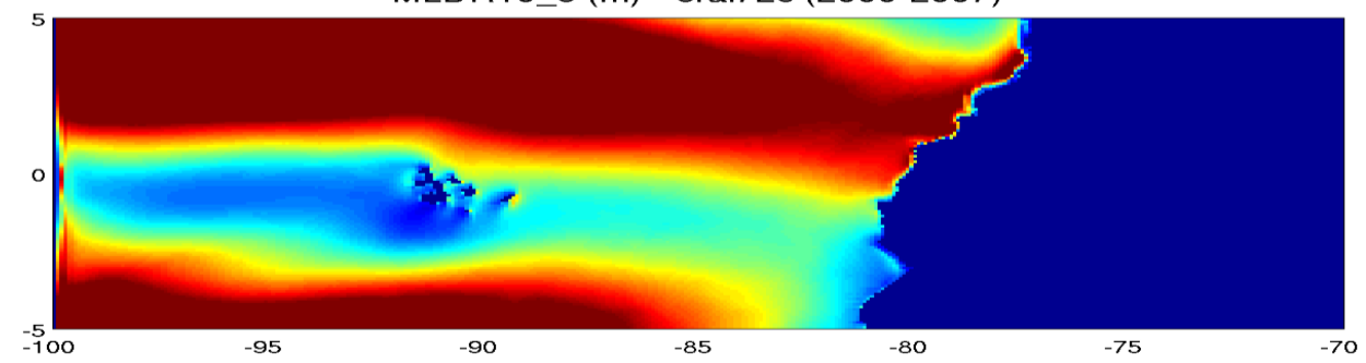
MLDR10_3 (m) - erai72c (2000-2007)
