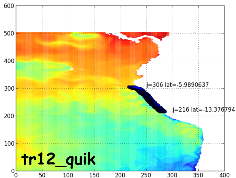
tr12_quik / 3240 particules: position initiale le 31 12 2008
